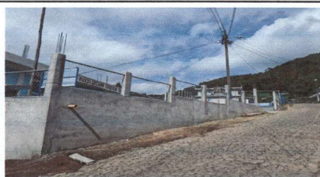
Foto 4: MUROS PERIMETRALES
